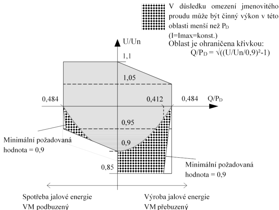
Obr. 2 Jalový výkon VM A1, A2 pro P=P_D
