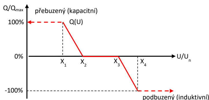
Obr. 20 Charakteristika funkce Q(U)
