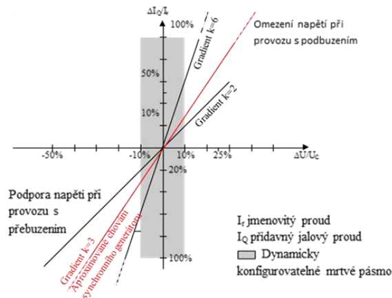
Obr. 13 Princip podpory napětí sítě zkratovým proudem nesynchronními VM
