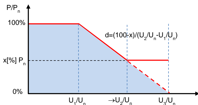
Obr. 19 Charakteristika funkce P(U)
