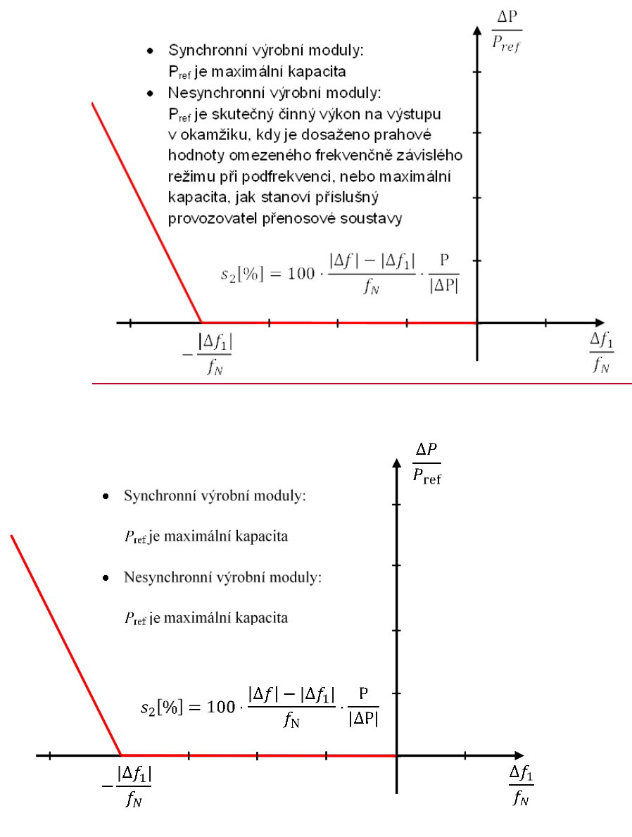
Obr. 16 Schopnost frekvenční odezvy činného výkonu u výrobních modulů v omezeném frekvenčně závislém režimu při podfrekvenci
