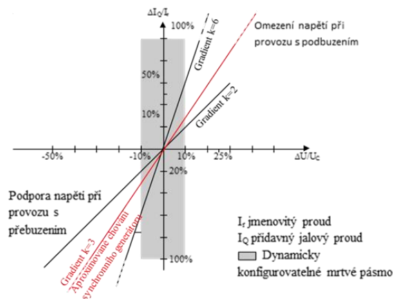
Obr. 13 Princip podpory napětí sítě zkratovým proudem nesynchronními VM
