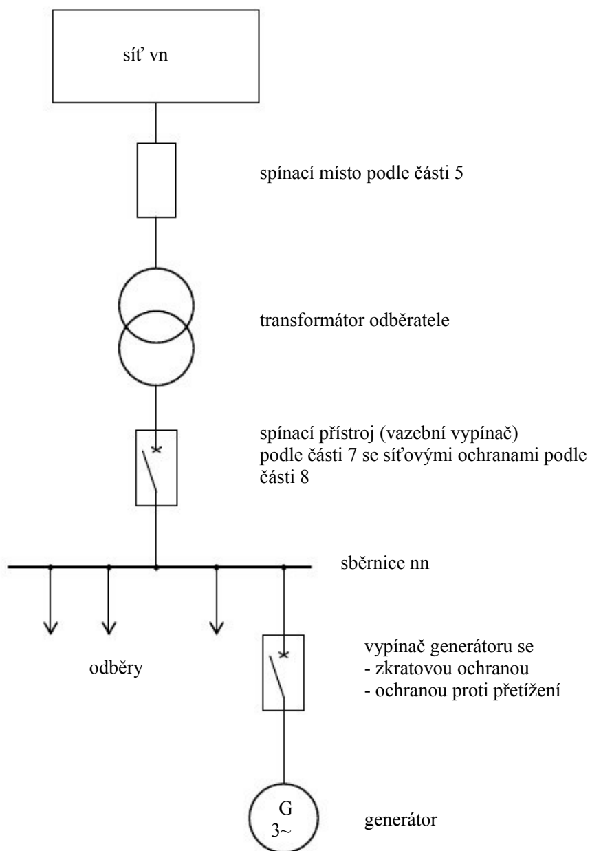
Příklad 5 Vlastní výroba v paralelním provozu se sítí s možností ostrovního provozu
