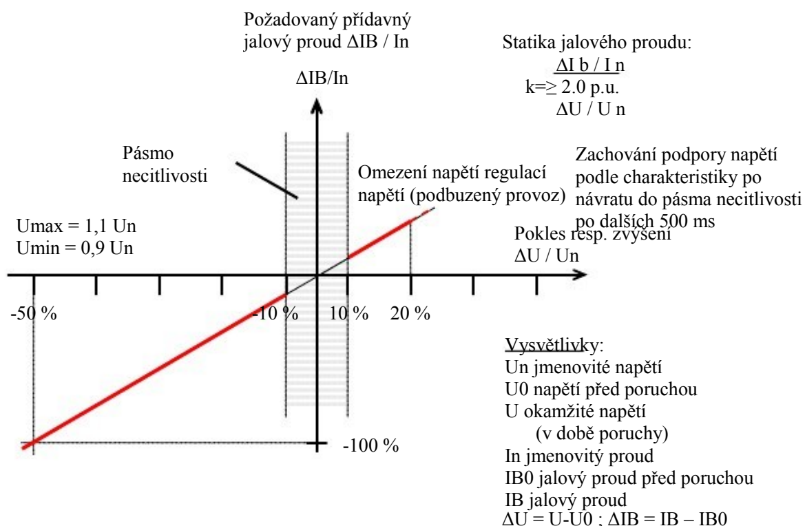
Obr. 3 Princip podpory napětí při poruchách v síti výrobny s obnovitelnými zdroji
