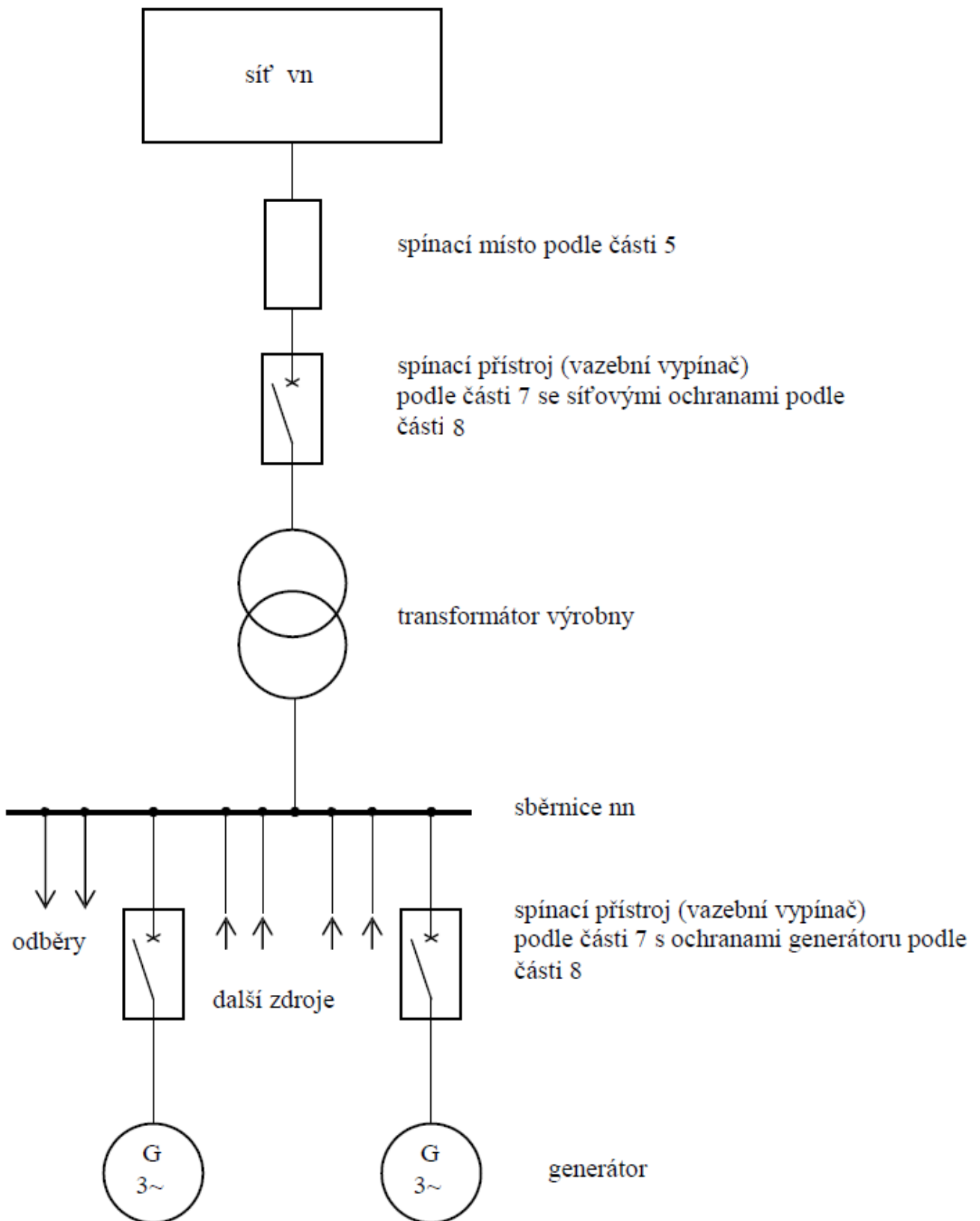
Příklad 6 Výrobna s více generátory v paralelním provozu se sítí s možností ostrovního
