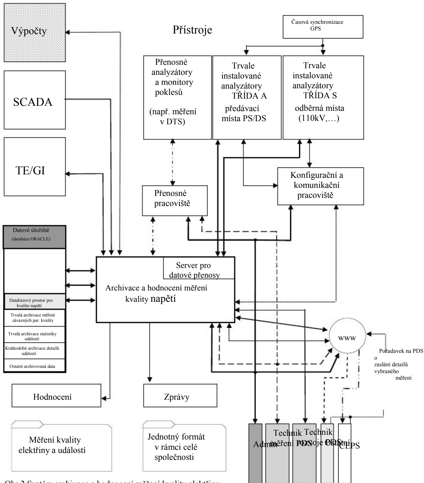
Obr.2 Systém archivace a hodnocení měření kvality elektřiny
