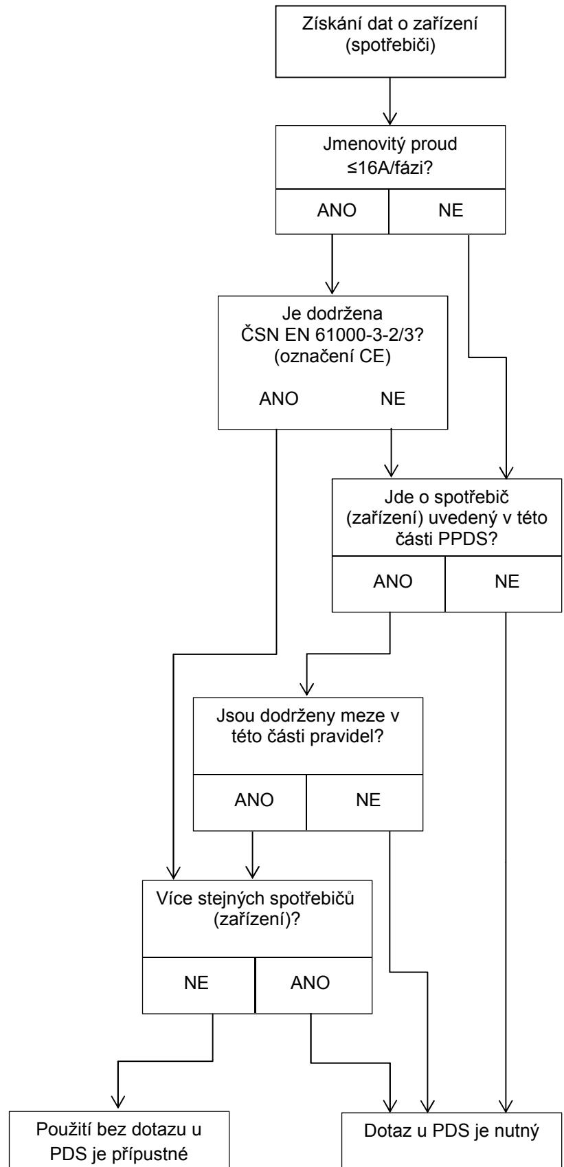
Obr. 1 Schéma po posuzování přístrojů/zařízení se zřetelem na elektromagnetickou kompatibilitu (EMC)
