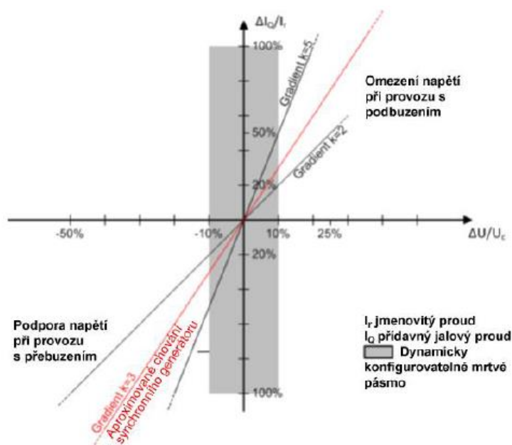
Obr. 4 Princip podpory napětí sítě při poruchách
