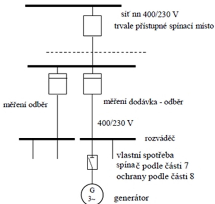
Příklad 1a Paralelně provozovaná výrobná v síti nn bez možnosti ostrovního provozu Společné připojení, možnost vykazat výrobu a částečně ji spotřebovat. Průběhové měření.
