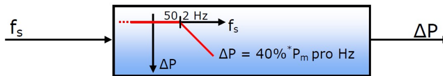
Obr. A Snížení činného výkonu obnovitelných zdrojů při nadfrekvenci
