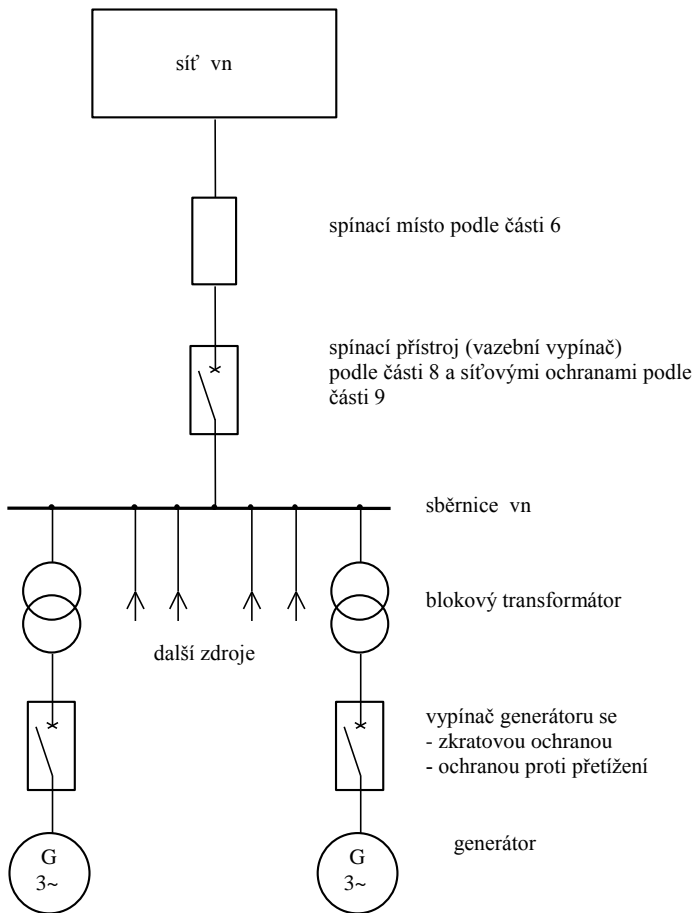
Příklad 8: Několik vlastních výroben v paralelním provozu se sítí bez možnosti ostrovního provozu, se sběrnici VN a centrálním vypínačem s ochranami
