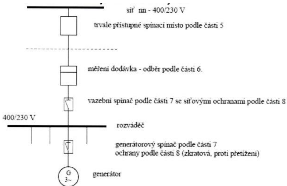
Příklad 1b: Paralelně provozovaná výrobná v síti NN bez možnosti ostrovního provozu. Celá výroba bez vlastní spotřeby dodaná do DS. Rozšíření stávajícího odběru o výrobu
