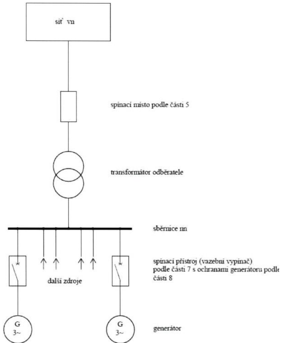
Příklad 4: Výrobna s více generátory v paralelním provozu se sítí bez možnosti ostrovního provozu
