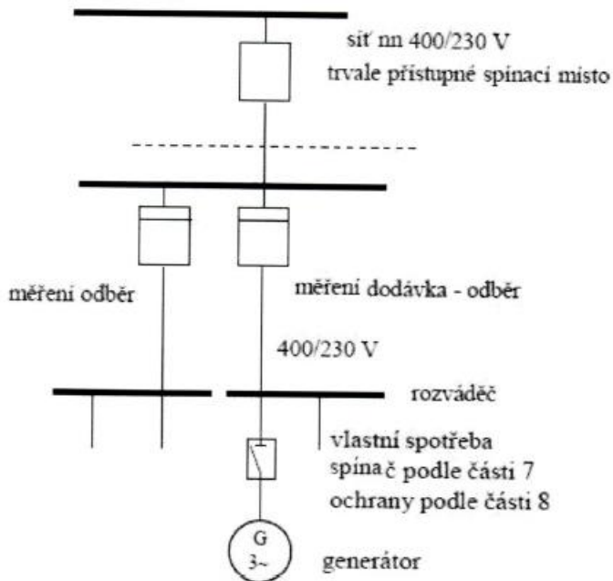
Příklad 1: Paralelně provozovaná výrobná v síti NN bez možnosti ostrovního Provozu
