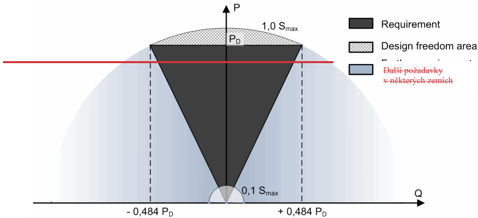
Obr.1 Požadavky na dodávku/odběr jalového výkonu při jmenovitém napětí
