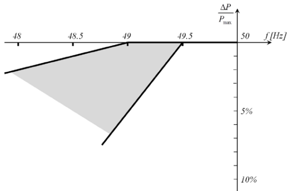
Obr. 15 Maximální snížení činného výkonu s klesajícím kmitočtem
