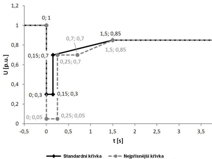
Obr. 38 Schopnost překlenutí poruchy synchronních VM A1, A2 a B1 (do 1 MW) přímo připojených generátorů
