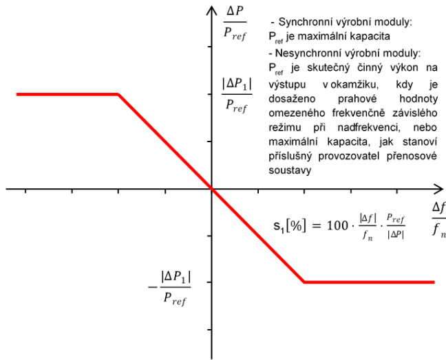
Obr. 17 Frekvenční odezva činného výkonu FSM
