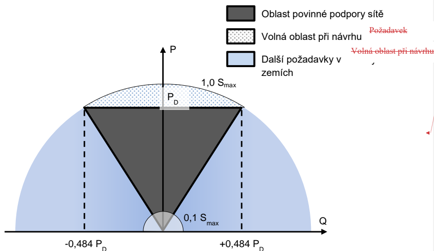
Obr. 1 Požadavky na dodávku/odběr jalového výkonu při U_n
