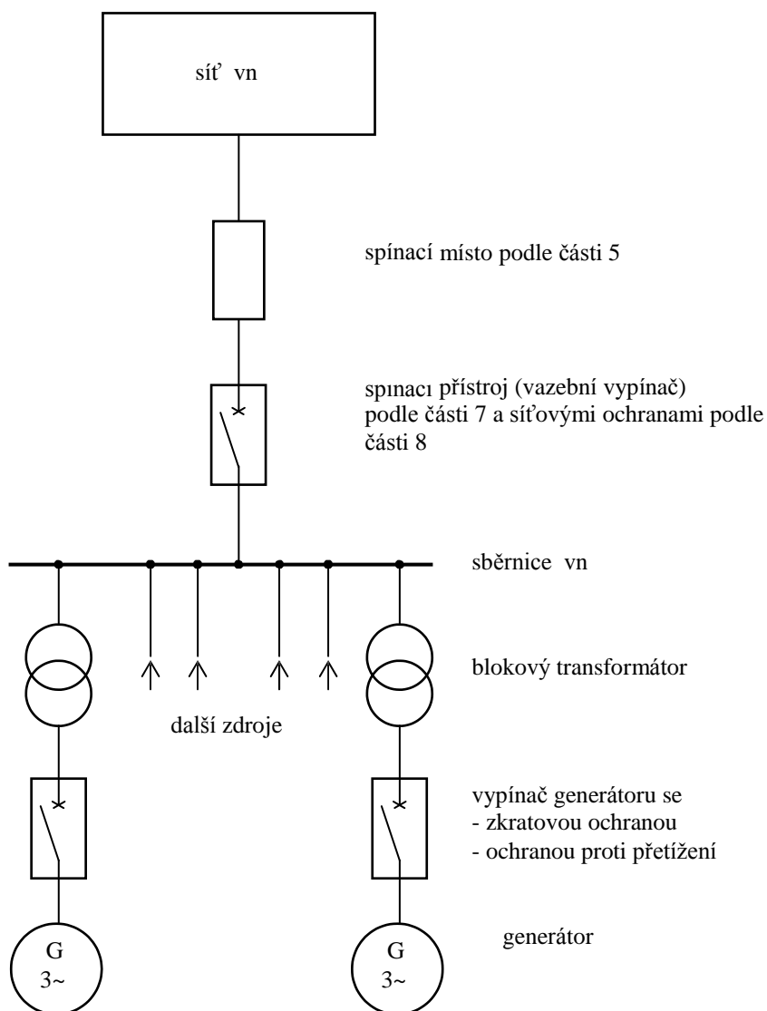
Příklad 8 Výrobna s více generátory v paralelním provozu se sítí bez možnosti ostrovního provozu, se sběrnici vn a centrálním vypínačem s ochranami
