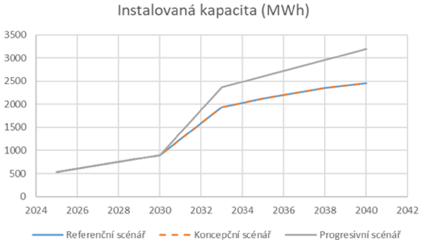
Graf 3 Předpokládaný vývoj instalované kapacity bateriové akumulace v ČR
