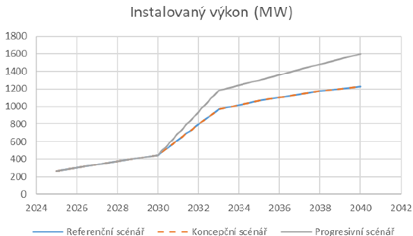
Graf 2 Předpokládaný vývoj instalovaného výkonu bateriové akumulace v ČR
