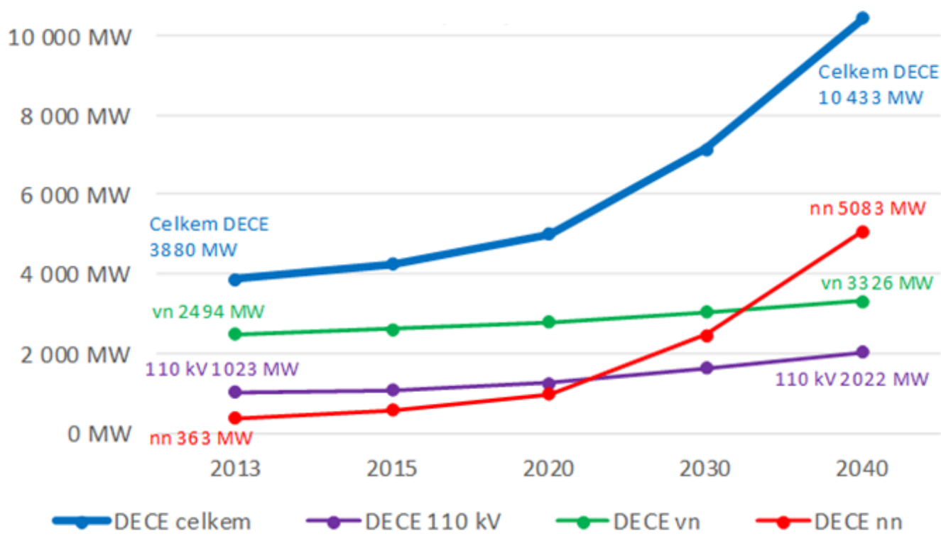
Graf 4 Vývoj celkového instalovaného výkonu decentrálních zdrojů podle NAP SG do roku 2040 podle napěťových hladin
