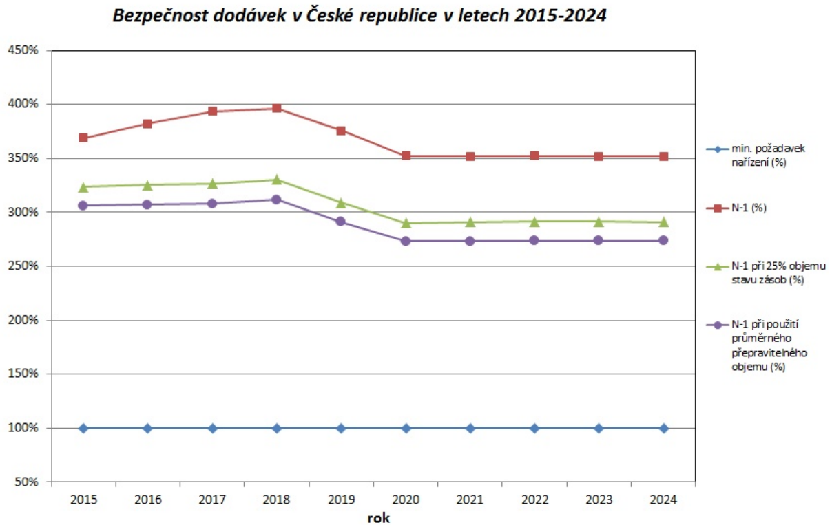
Graf 14 Bezpečnost dodávek v České republice v letech 2015-2024
