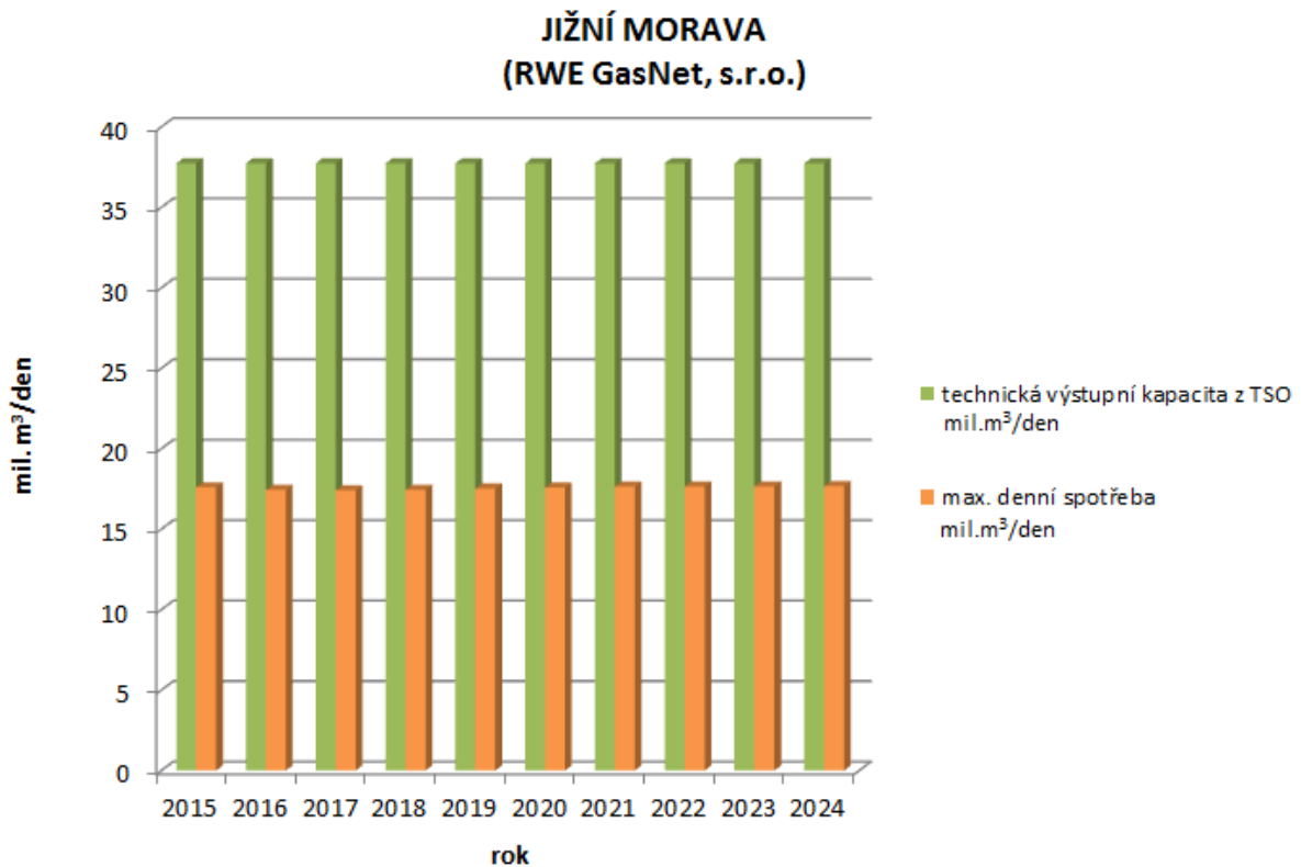
Graf 9 Přiměřenost výstupní kapacity a vývoj maximální denní spotřeby plynu v regionu jižní Morava (RWE GasNet, s.r.o., dříve JMP Net, s.r.o.)
