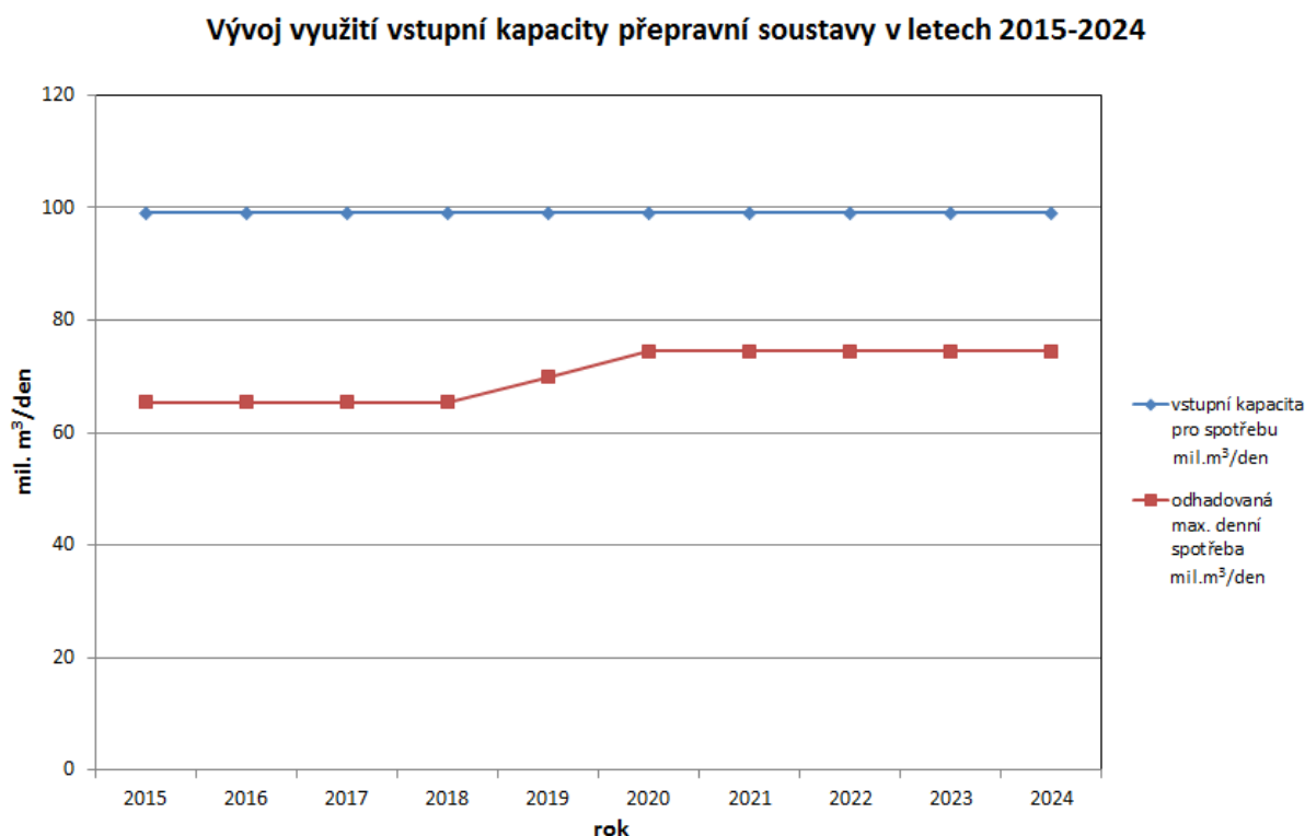
Graf 4 Vývoj využití vstupní kapacity přepravní soustavy v letech 2015-2024
