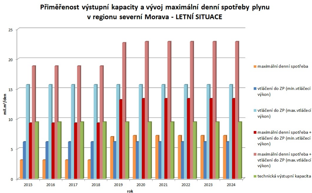
Graf 10 Přiměřenost výstupní kapacity a vývoj maximální denní spotřeby plynu v regionu severní Morava – letní situace
