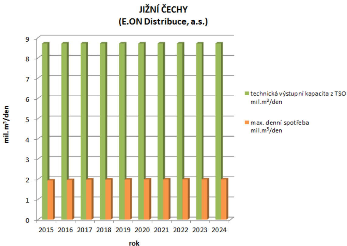
Graf 5 Přiměřenost výstupní kapacity a vývoj maximální denní spotřeby plynu v regionu jižní Čechy (E.ON Distribuce, a.s.)
