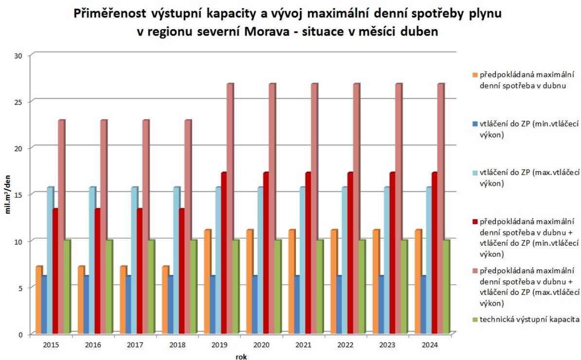
Graf 12 Přiměřenost výstupní kapacity a vývoj maximální denní spotřeby plynu v regionu severní Morava – situace v měsíci duben
