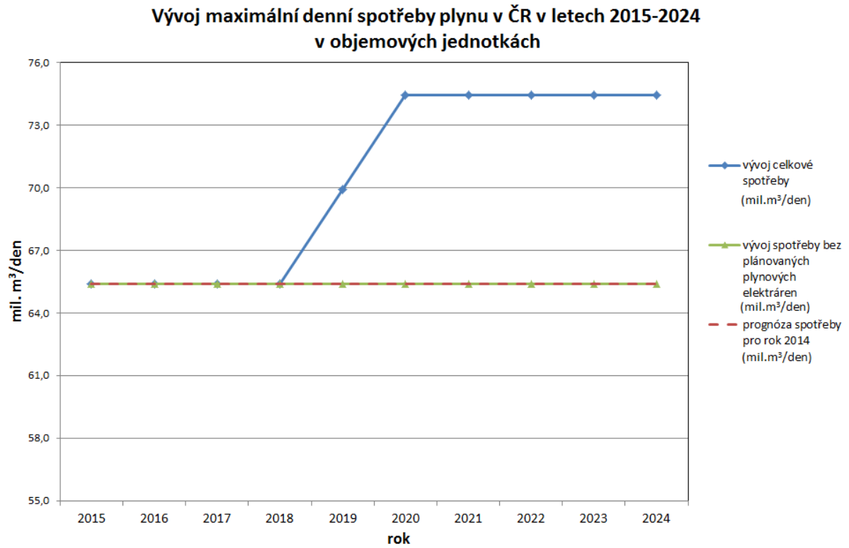
Graf 3 Vývoj maximální denní spotřeby plynu v České republice v letech 2015-2024 v objemových jednotkách
