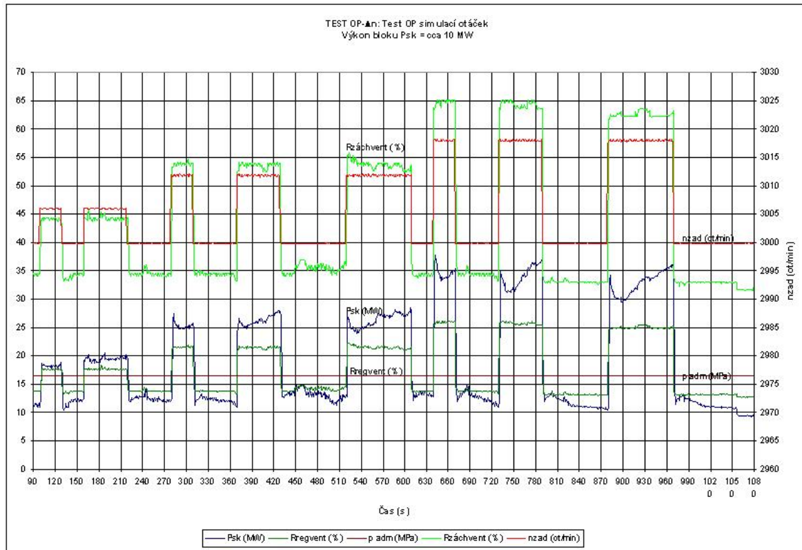
Obr. č. 32 Příklad TEST (OP) – Δn – skokové změny otáček
