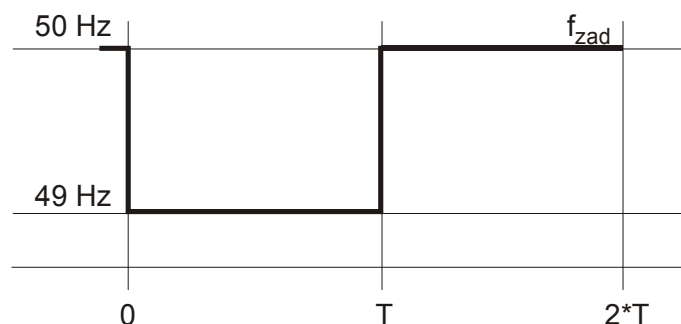
Obr. č. 28 TEST 1 (OP)-VE – Příklad simulované změny f_{zad} na hladině P_{maxROP}
