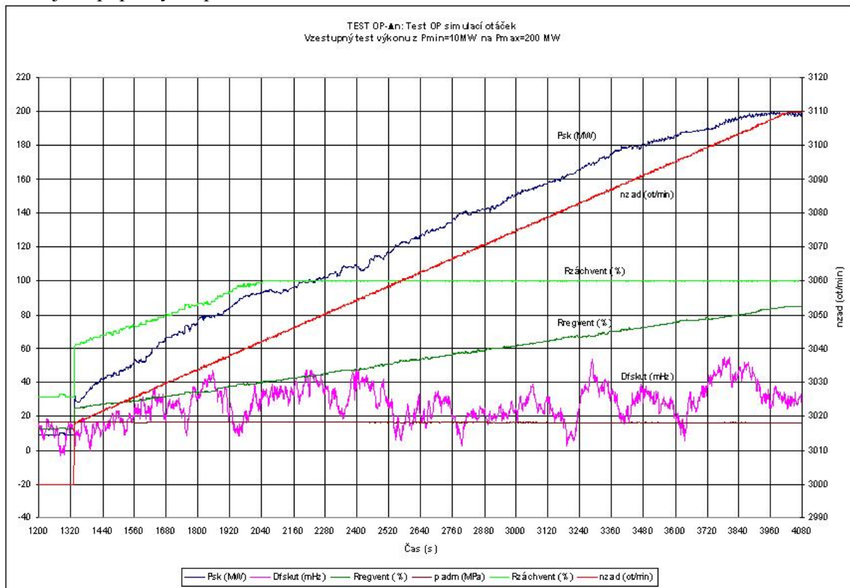
Obr. č. 31 Příklad TEST (OP) – \Delta n – plynulé změny otáček
