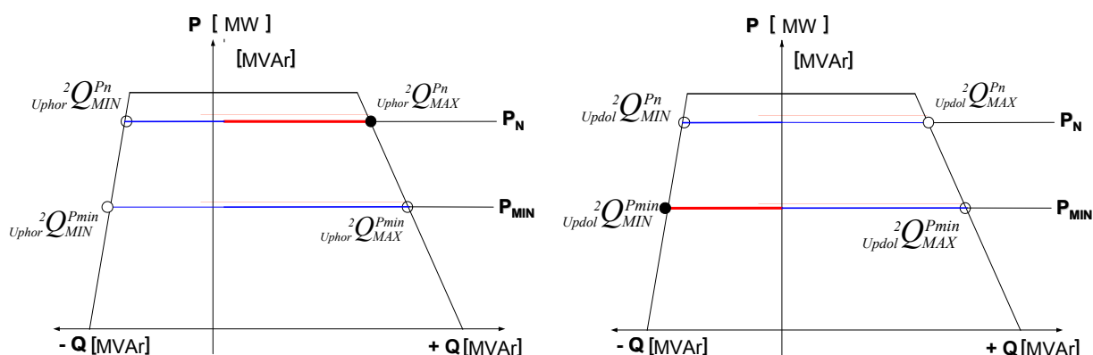
Obr. č. 20 TEST (SRUQ)-ON - Naměřené hodnoty v PQ diagramu bloku při U_{phor} a U_{pdol}
