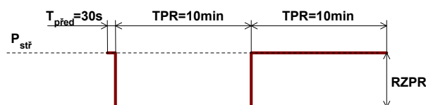
Obr. č. 4 TEST (PR)-Δf - Průběh požadovaného činného výkonu pro jednotlivá měření
