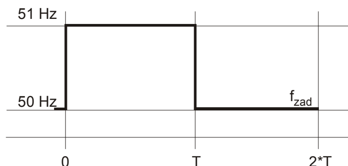
Obr. č. 29 TEST 1 (OP)-VE – Příklad simulované změny f_{zad} na hladině P_{minROP}
