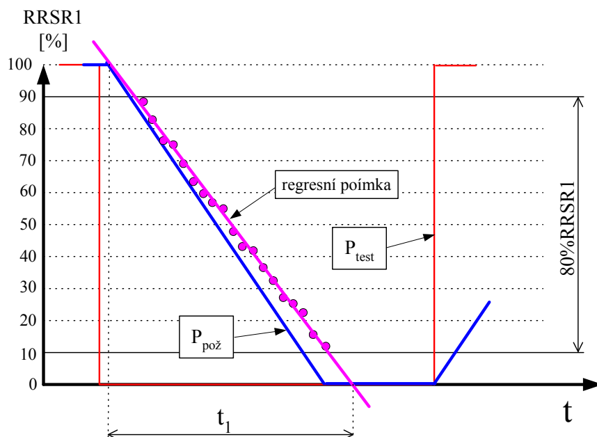
Obr. č. 13 TEST SR-AP - Konstrukce regresní přímky pro výpočet CSR_{skut}
