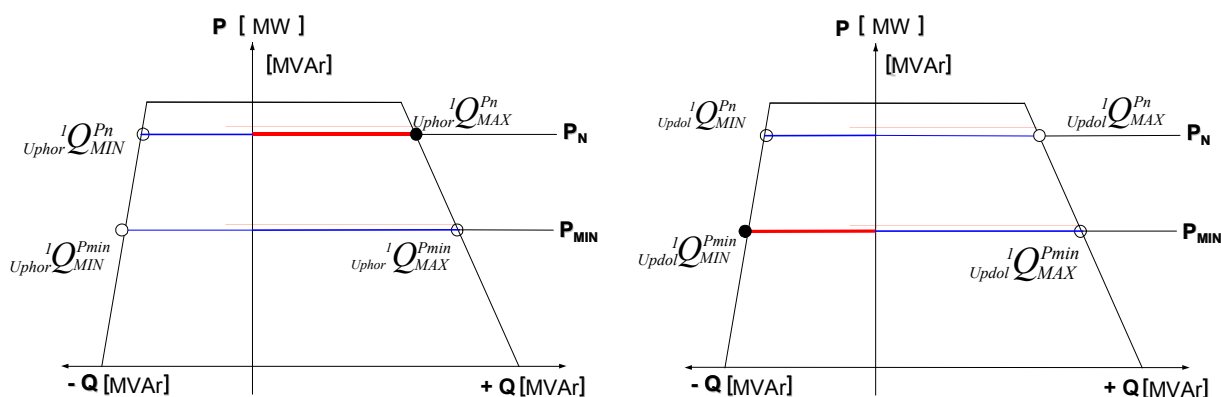
Obr. č. 19 TEST (SRUQ)-OFF - Naměřené hodnoty v PQ diagramu bloku při U_{phor} a U_{pdol}
