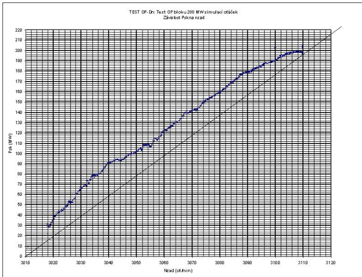
Obr. č. 33 Příklad TEST (OP) – Δn – plynulé změny otáček
