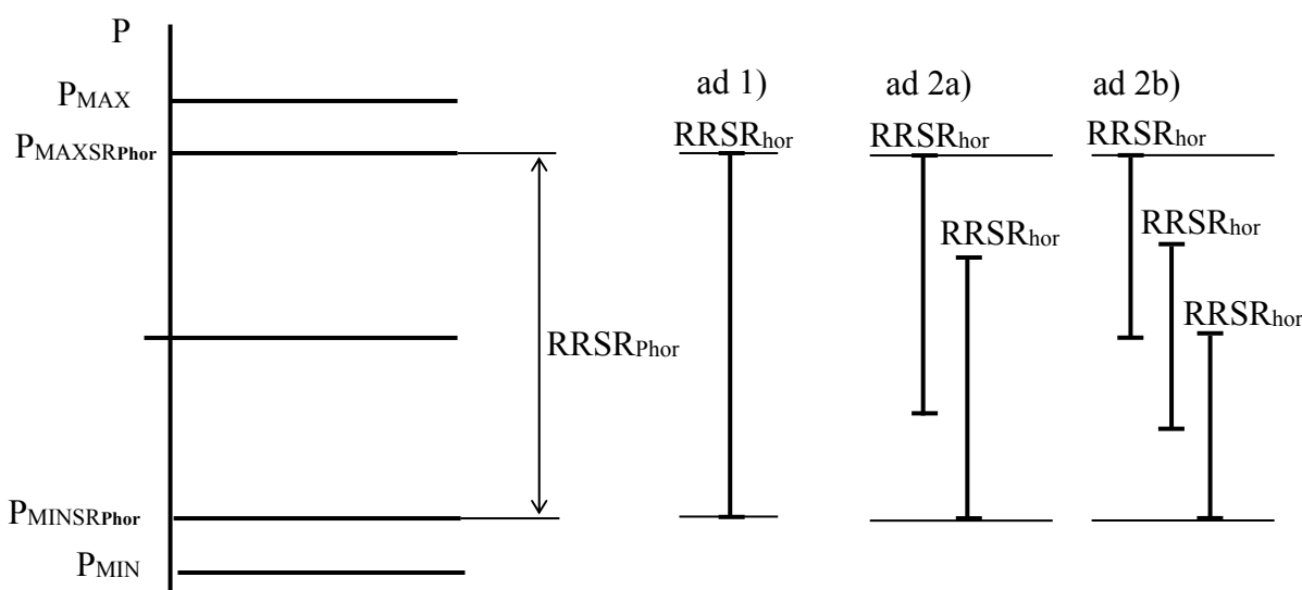
Obr. č. 9 Volba mezi jednotlivých RRSR při certifikaci - příklad pro horní provozní pásmo - index i = \text{hor} (stejnou formou je případně volba prováděna i pro RRSR_{Pstř} a RRSR_{Pdol} ).
