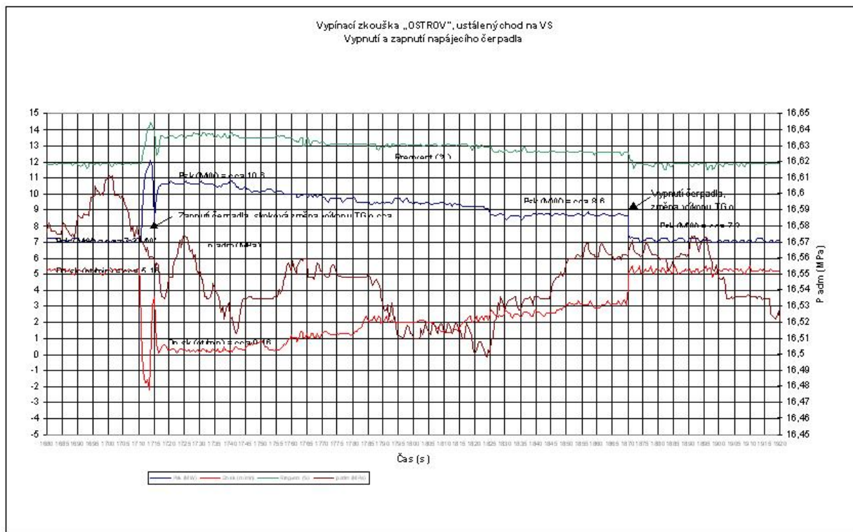
Obr. č. 30 Příklad TEST (OP) – ostrov – změna vlastní spotřeby
