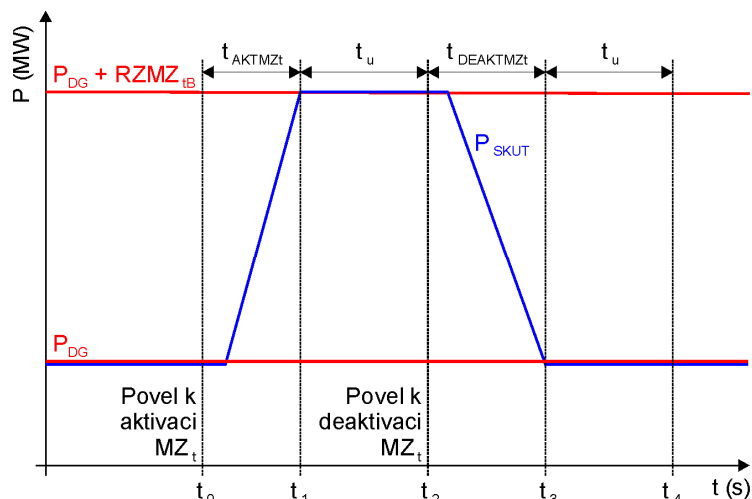
Obr. č. 17 Průběh certifikačního testu MZ_{t_B}
