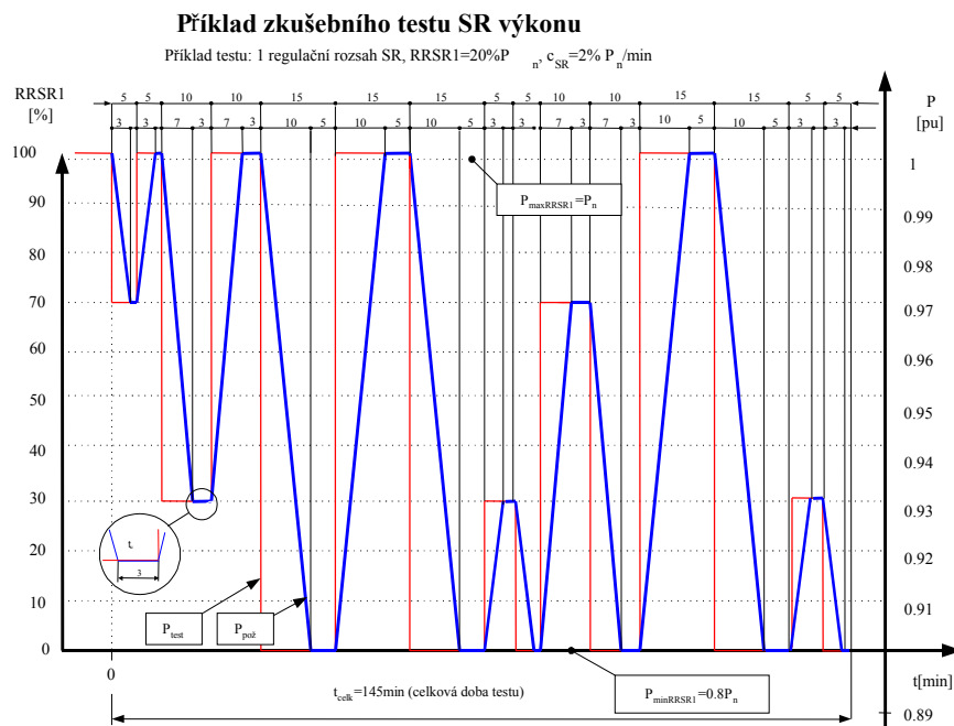
Obr. č. 14 P test – příklad
