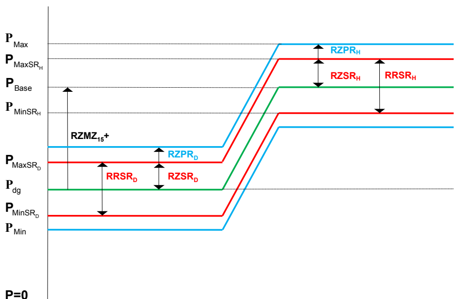
Obr.1.1 Příklad typového rozložení výkonových záloh na elektrárenském bloku pro PpS, v případě symetrické SR a při užití MZ_{15+} (analogicky pro MZ_{15-} )
