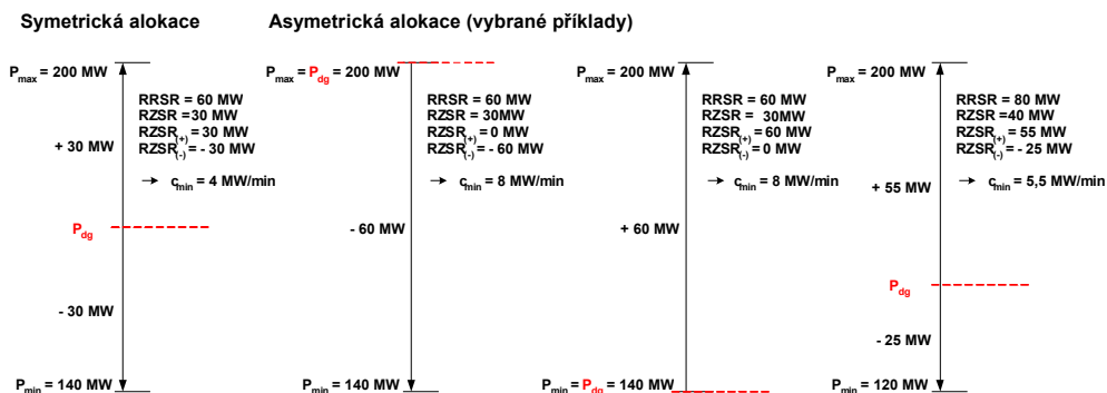
Obr.1.2 Příklad regulačních záloh a regulačních rozsahů na elektrárněnských blocích pro symetrickou a asymetrickou alokaci PpS SR
