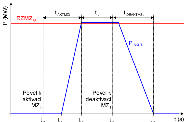
Obr. č. 16 Průběh certifikačního testu MZ_{t_A}
