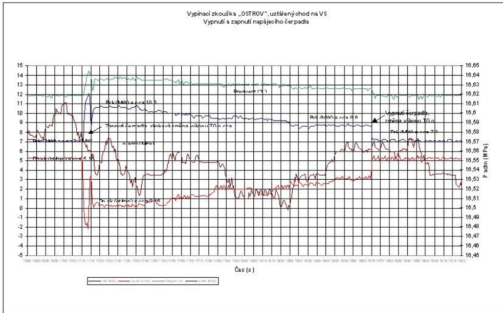
Obr. č. 32 Příklad TEST (OP) – ostrov – změna vlastní spotřeby
