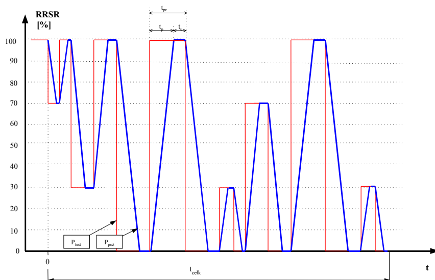
Obr. č. 11 TEST SR-AP - Tvar testovacího signálu
