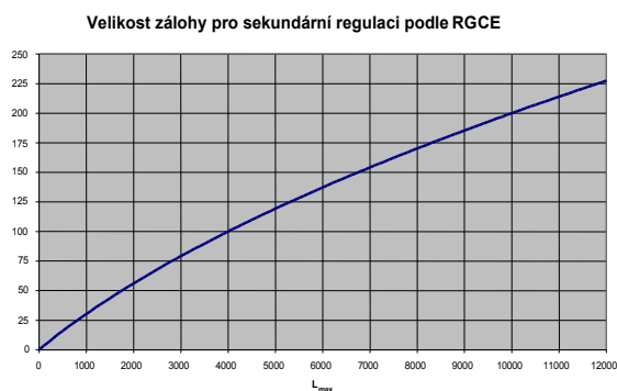
Obr. 2.1 Velikost zálohy pro sekundární regulaci podle RGCE
