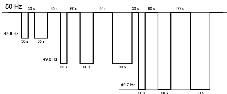
Obr. č. 26 TEST (OP)- \Delta n – Příklad průběhu testovacího signálu n_{zad} nebo f_{zad} pro P_{hMĚŘ}
