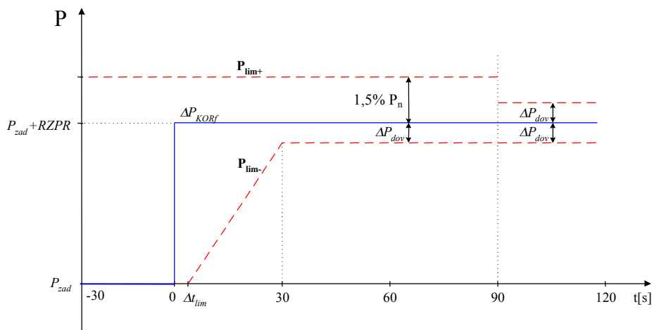
Obr. č. 5 TEST (PR)- \Delta f - Požadavky na průběh skokové změny činného výkonu
