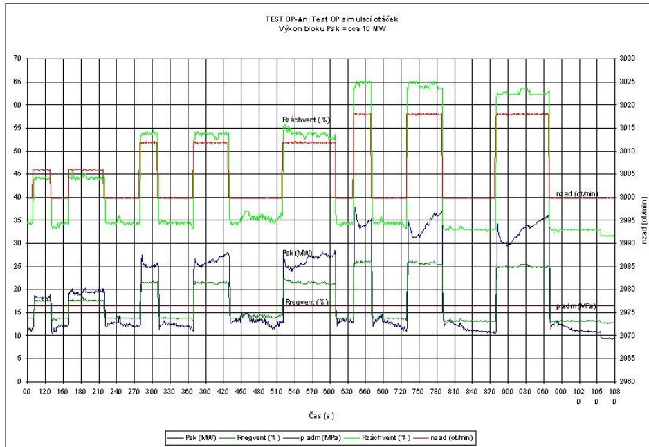
Obr. č. 34 Příklad TEST (OP) – \Delta n – skokové změny otáček
