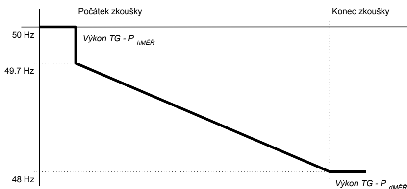
Obr. č. 29 TEST (OP)- \Delta n – Příklad simulované plynulé změny otáček – sestupný test
