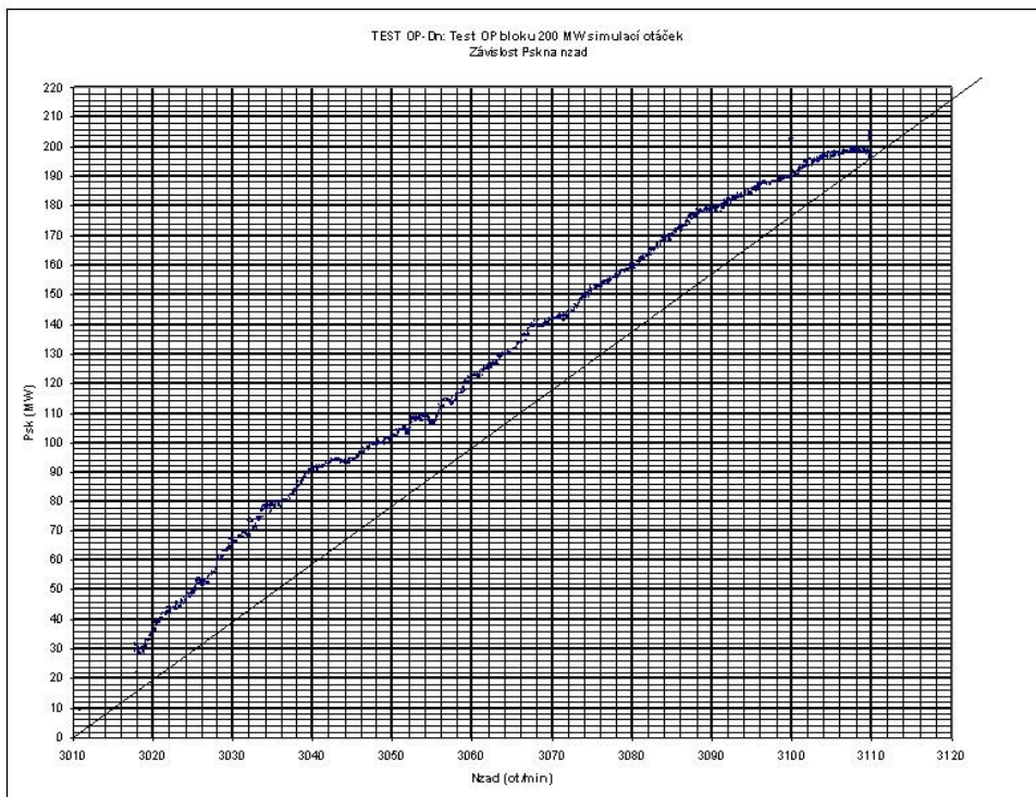
Obr. č. 35 Příklad TEST (OP) – \Delta n – plynulé změny otáček
