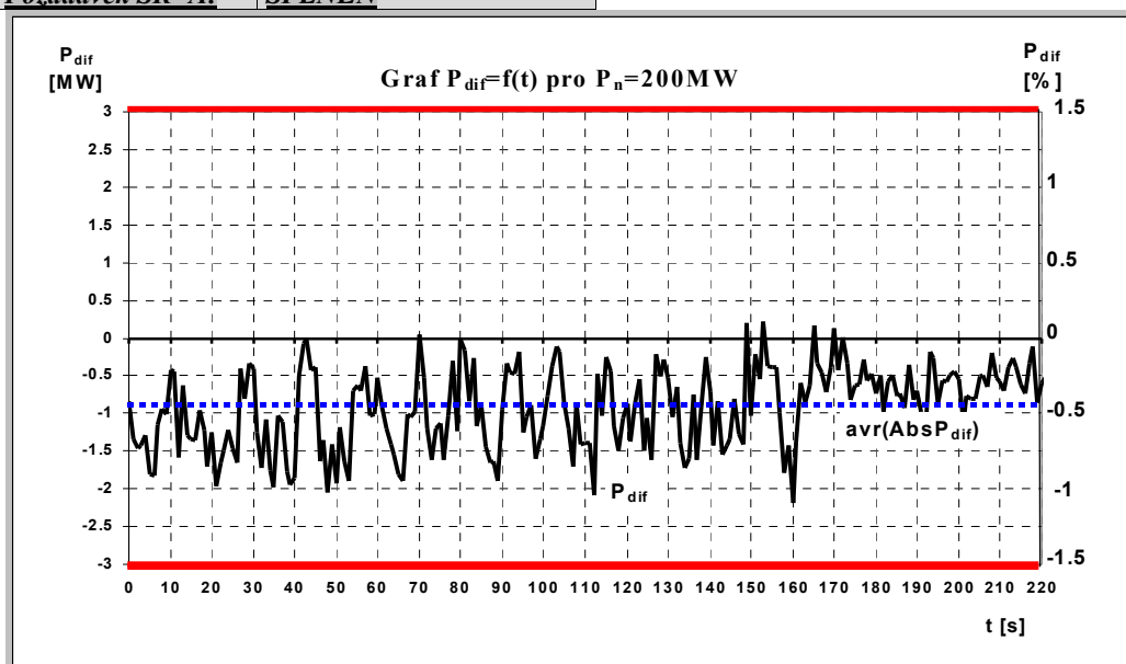
Obr. č. 15 Závislost P_{dif}=f(t)
