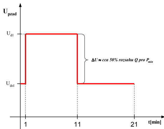
Obr. č. 23 TEST (SRUQ)-AU-blok - Zadané napětí v pilotním uzlu při podbuzení
