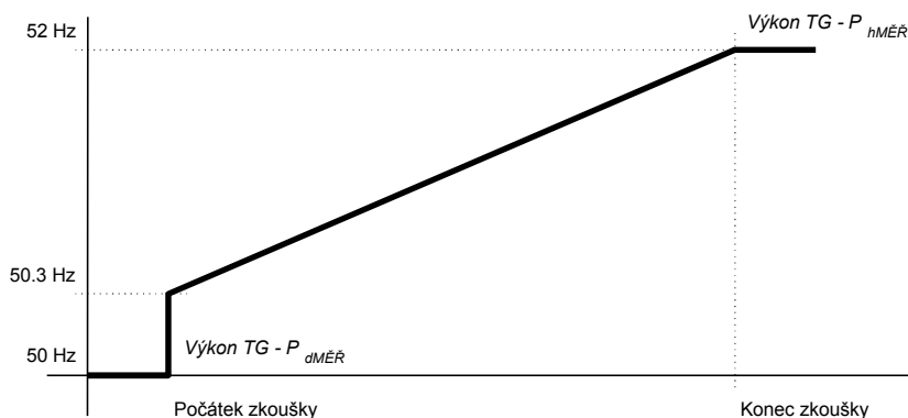
Obr. č. 28 TEST (OP)-An – Příklad simulované plynulé změny otáček – vzestupný test
