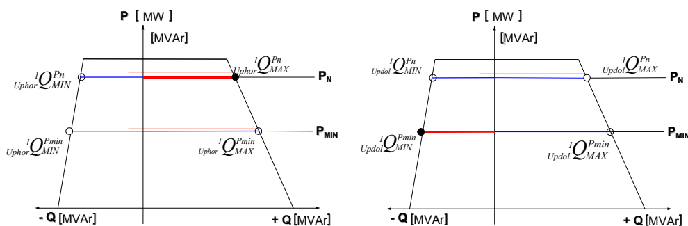
Obr. č. 21 TEST (SRUQ)-OFF - Naměřené hodnoty v PQ diagramu bloku při U_{phor} a U_{pdoi}
