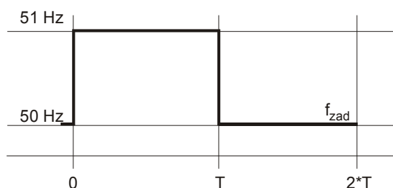
Obr. č. 31 TEST 1 (OP)-VE – Příklad simulované změny f_{\text{zad}} na hladině P_{\min\text{ROP}}
