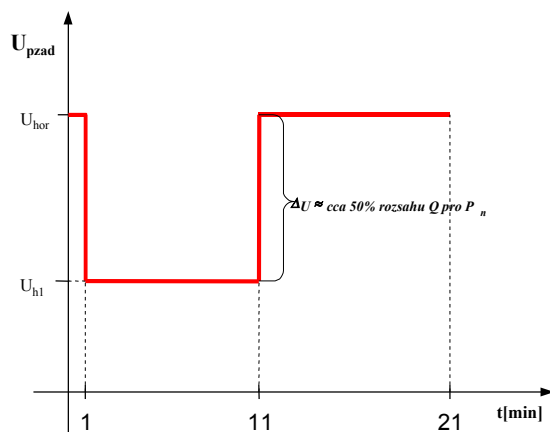
Obr. č. 24 TEST (SRUQ)-AU-blok - Zadané napětí v pilotním uzlu při přebuzení
