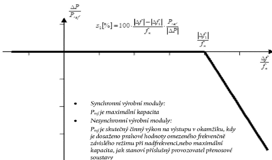
Obr. 1 Diagram LFSM-O
